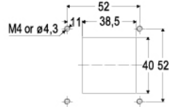
カタログ図面
