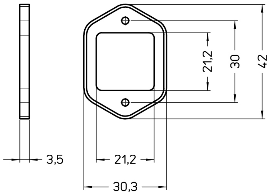
カタログ図面
