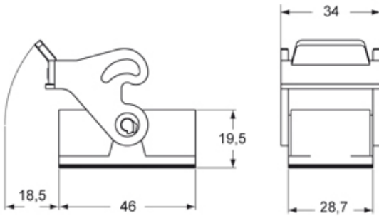
カタログ図面
