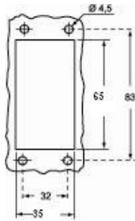
カタログ図面
