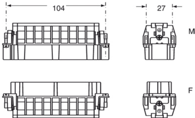
カタログ図面
