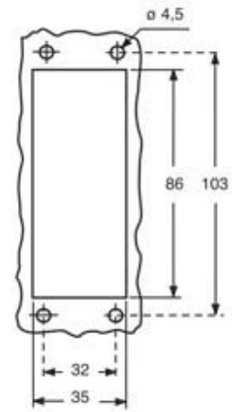
カタログ図面
