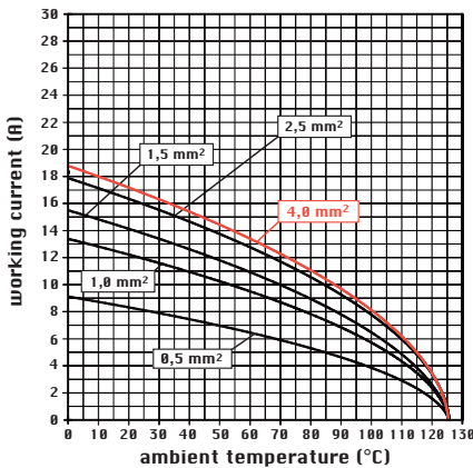
diagram JSE 48 poles
